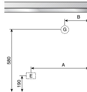
VISTA POSTERIORE PD70 - PT100 - PT110
