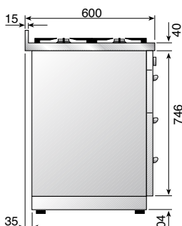
VISTA LATERALE PD70 - PT100 - PT110
