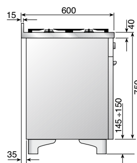
VISTA LATERALE QDC (CLASSICO)
